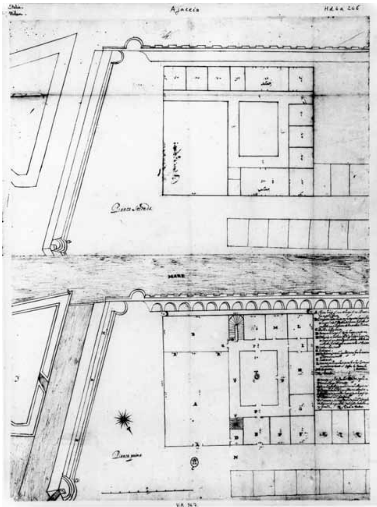
1. Ajaccio, Plan Nr. 1 (Ausschnitt).
