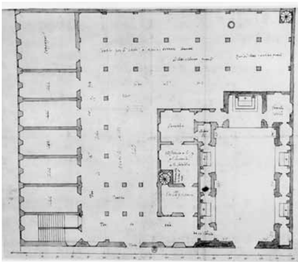
2. Ajaccio, Plan Nr. 2.
