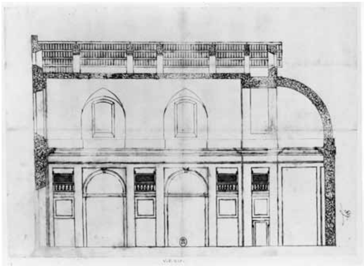
6. Ajaccio, Plan Nr. 5 (Längsschnitt der Kirche).
